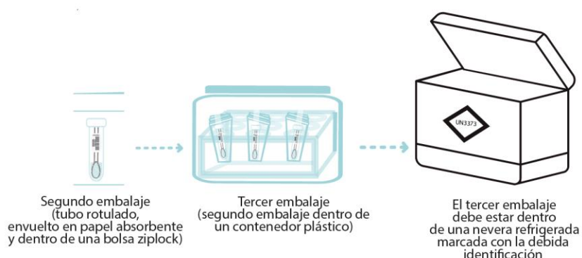
Figura 3. Triple embalaje para transporte de muestras. Elaboración propia
